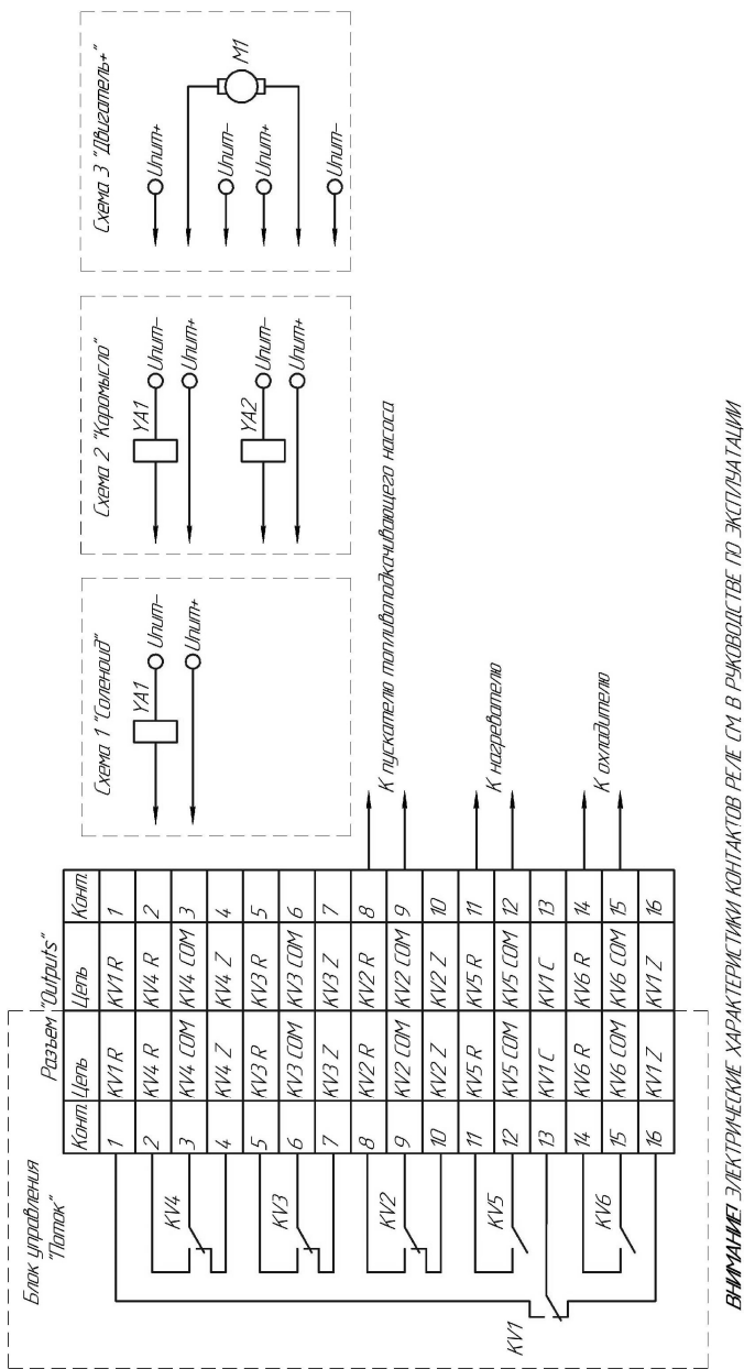
Рисунок А.1 – Распайка разъема "Outputs". Пример подключения шторки и системы кондиционирования
